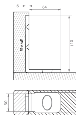
DOOR JAM BRACKET DETAIL
