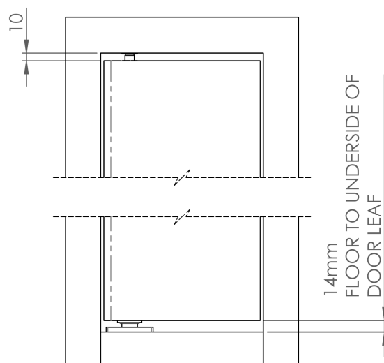
ELEVATION - DOOR
